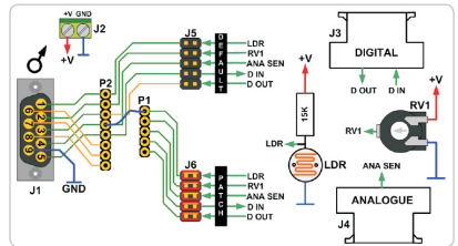
Bild 4 - Schaltung des gepatchten Sensor-Bords
